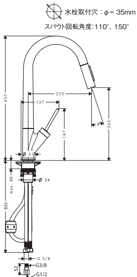
31815004 フォーカス シングルレバーキッチン混合水栓 引出式 ハイสบアウト 240 (シャワー切替)
